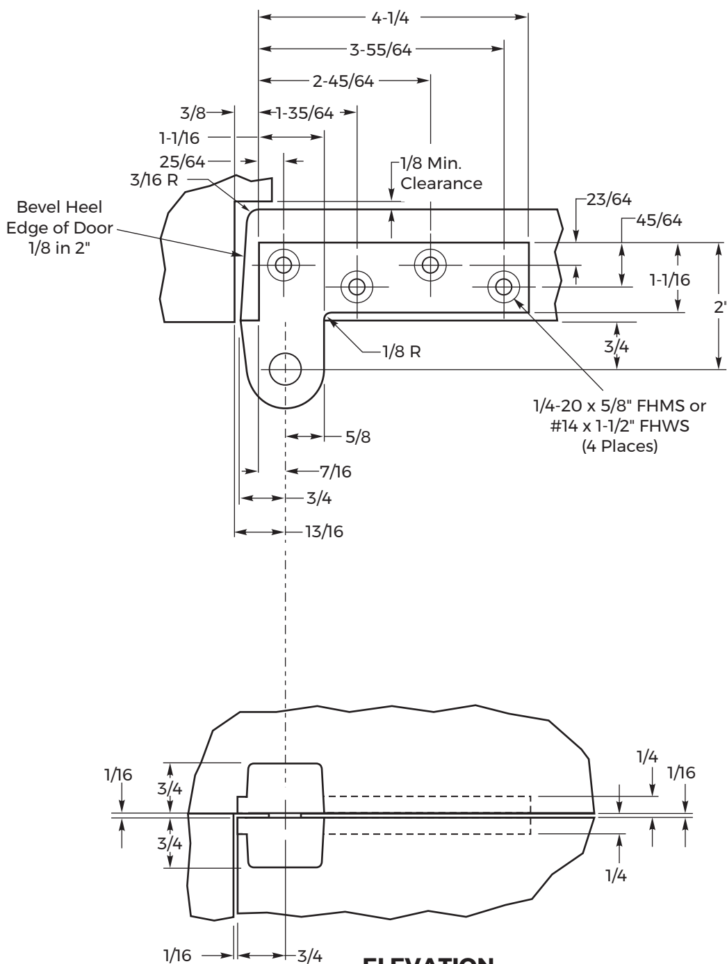
ELEVATION
