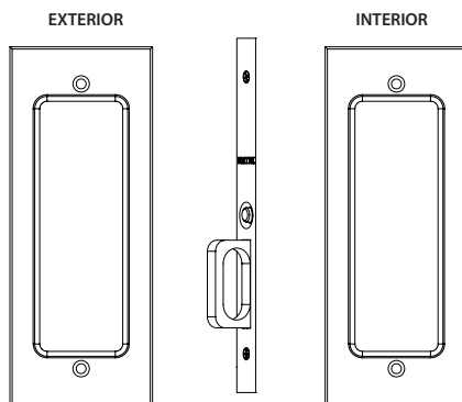
Passage Door Mortise Lock
