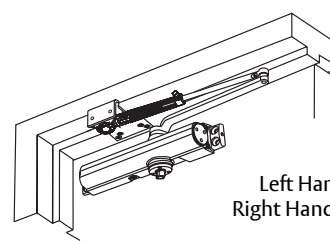
Right Hand Door - RH Left Hand Reverse - LHR
