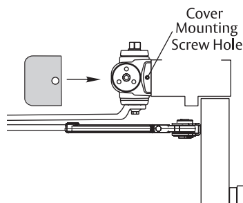
Top Jamb Mount
