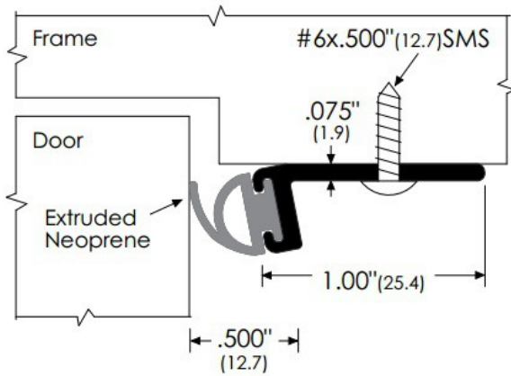
Door Gasket:
