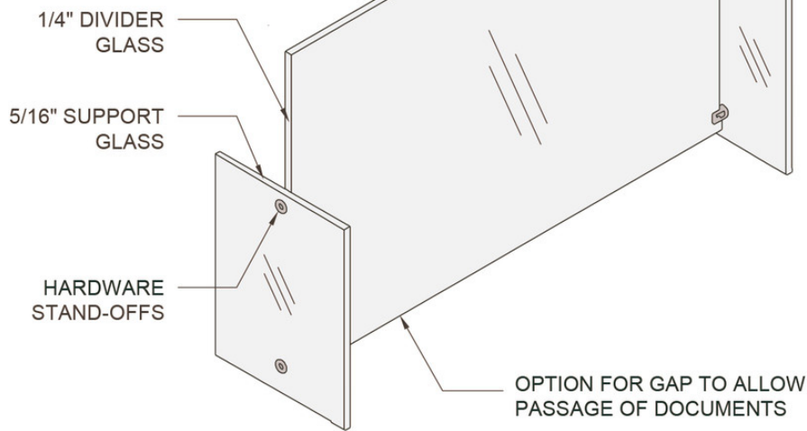
TYP. ISOMETRIC
