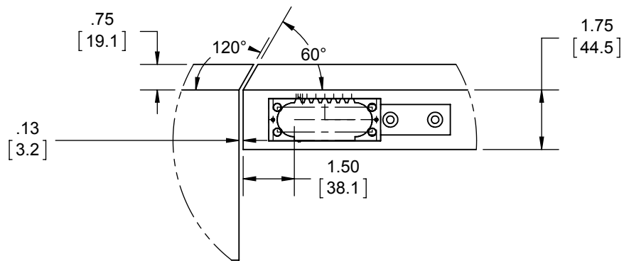
DETAIL A 1 : 4
