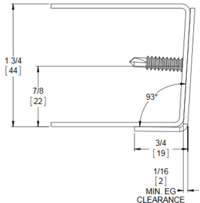
Bevel edge door
