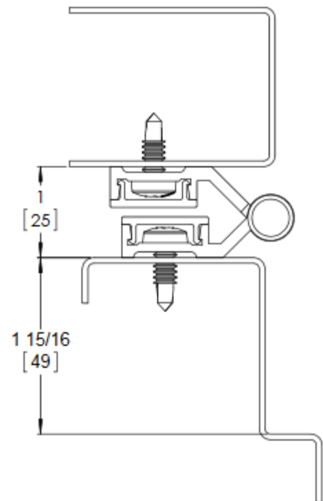
Door Open 180°
