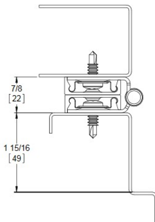
Door Open 180°
