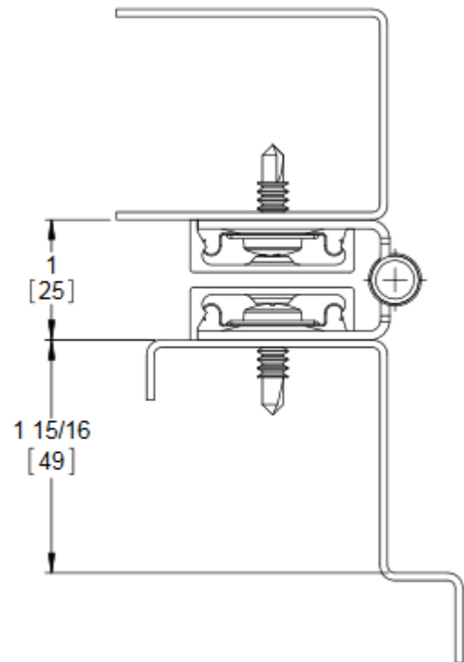
Door Open 180°
