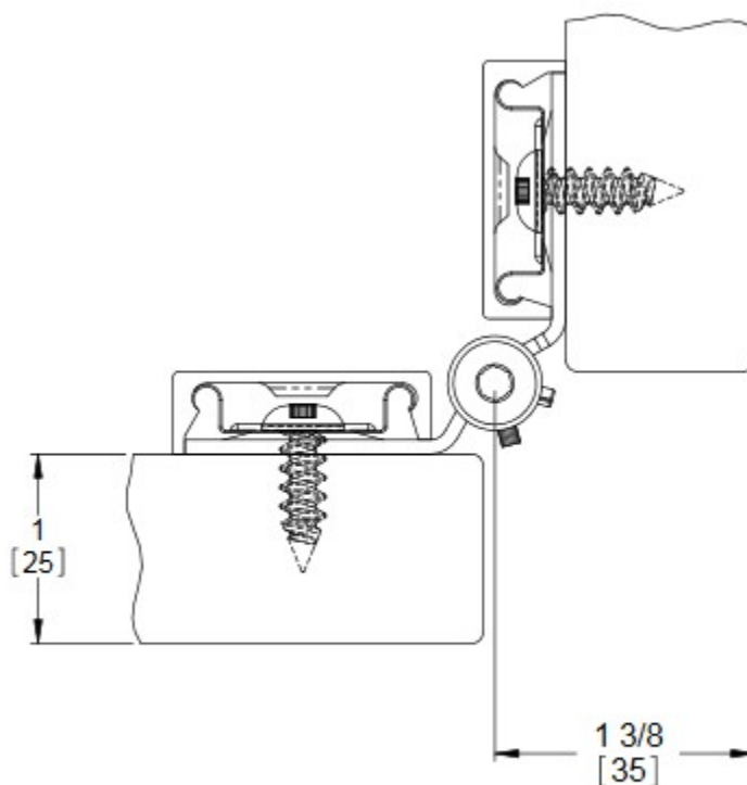
Door Open 90°
