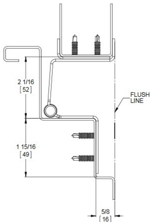
Door Open 90°
