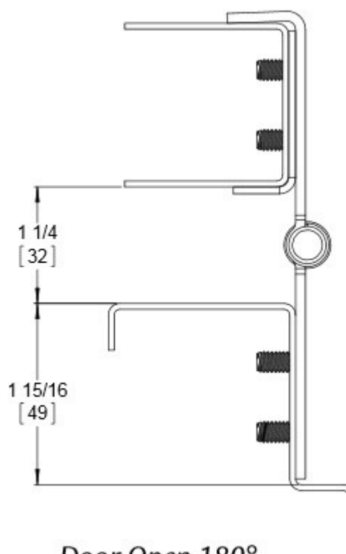
Door Open 180°
