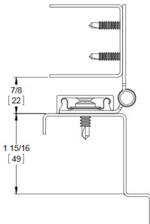
Door Open 180°
